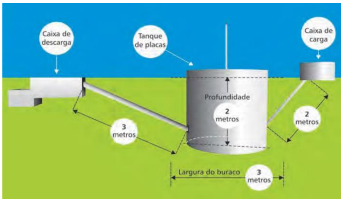
FIGURA 1 – Estrutura de montagem de um biodigestor indiano adaptado às condições sertanejas
