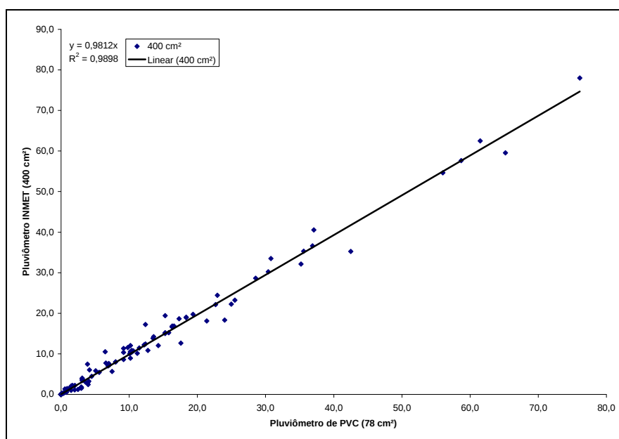
Figura 12 – Comparação do pluviômetro de padrão e do pluviômetro de PVC Organizador: SOUSA, R. R., 2016.
