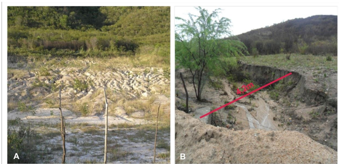
Figura 05 – A: Grande número de sucros e ravinas em antiga área de extração de areia. B: Voçoroca em estágio avançado, encosta próxima a área de extração Foto: Leandro Pereira, 2012.
