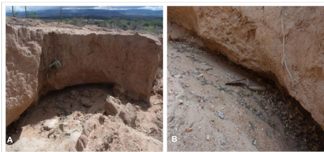
Figura 07 – A: Processo evolutivo de voçoroca a partir do escoamento subsuperficial. B: Microcanaís formados no interior da voçoroca por efeito do escoamento subsuperficial. Foto: Leandro Pereira, 2012.
