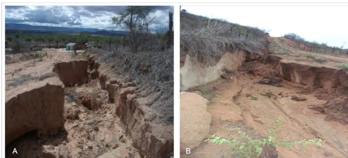
Figura 08 – A: Voçoroca vista de cima para baixo, em período de estiagem. B: Voçoroca vista de baixo para cima, logo após evento chuvoso. Foto: Leandro Pereira, 2012.
