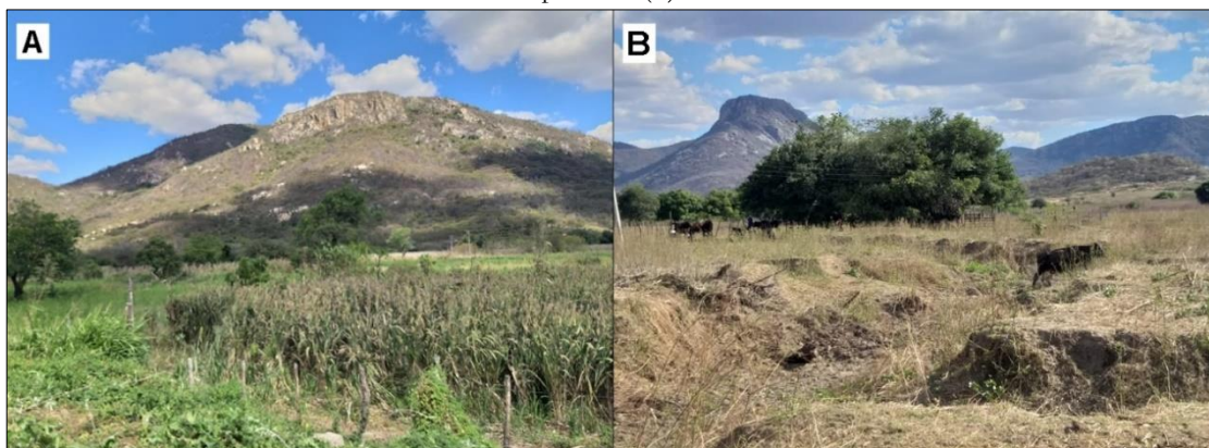
Figura 4 – Planície do rio Figueiredo com atividades de agricultura (A); Planície do riacho Amparo com pecuária (B).
