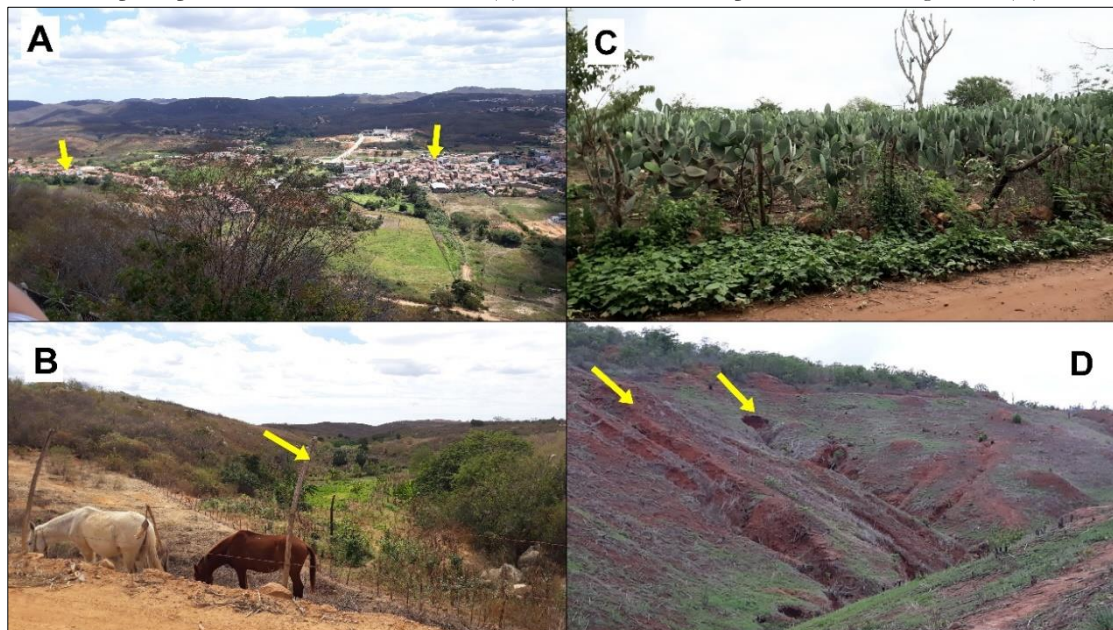
Figura 2 – Sede municipal de Pereiro no topo serrano (A); Cultura permanente de palma forrageira (B); Vale ocupado por atividades de subsistência (C); Erosão ocasionada pela retirada da vegetação (D).
