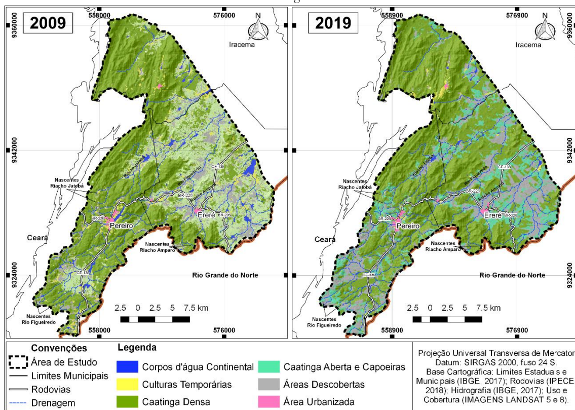
Figura 6 – Uso e Cobertura Multitemporal das Áreas de Nascentes do Alto Curso da Sub-bacia Hidrográfica do Rio Figueiredo.
