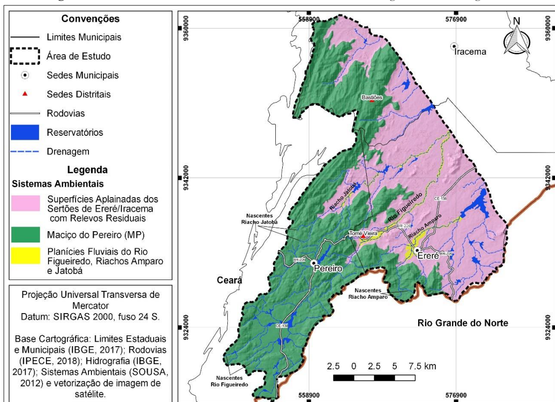
Figura 5 – Sistemas Ambientais do Alto Curso da Sub-bacia Hidrográfica do Rio Figueiredo.
