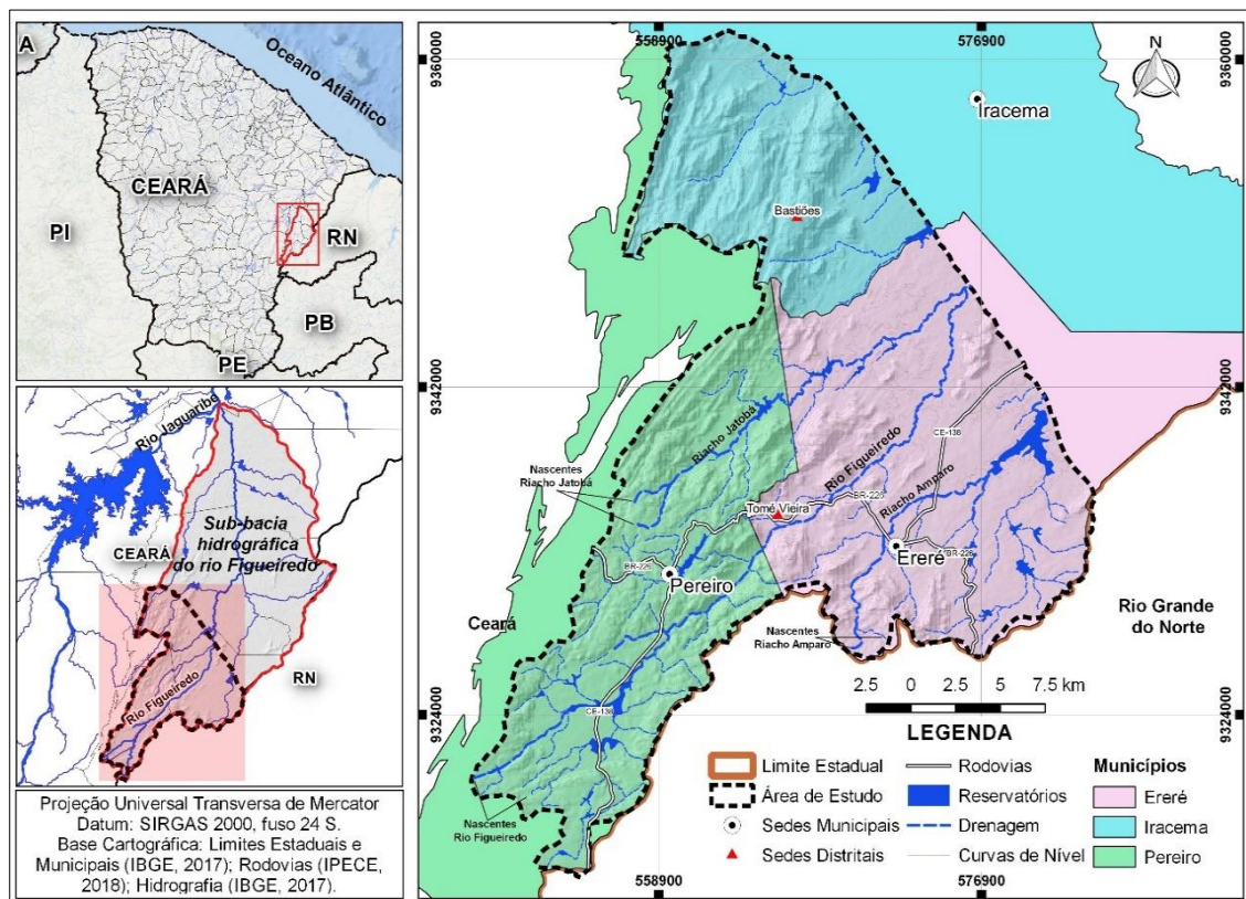
Figure 1 – Localização das Áreas de Nascentes do Alto curso da Sub-bacia Hidrográfica do Rio Figueiredo, Ceará.
