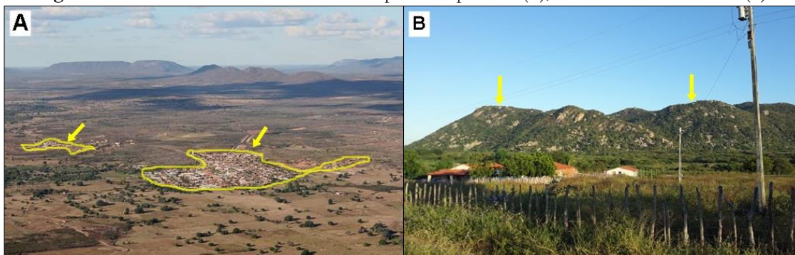
Figura 3 – Sede urbana de Ereré em meio a Superfície Aplainada (A); Relevo residual em Ereré (B).
