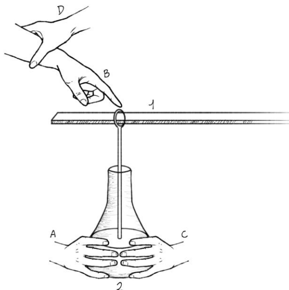
Figura 4 – Representação do primeiro arranjo
