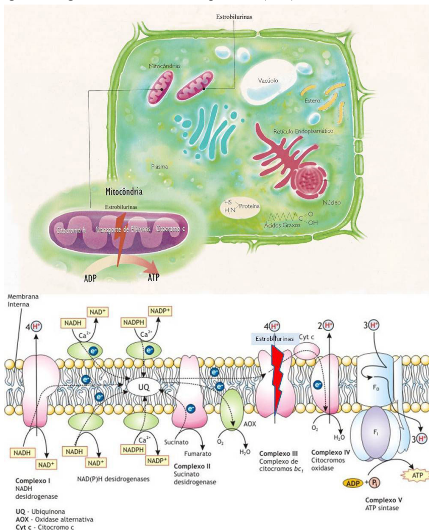
Figura 2. Célula fúngica, com detalhe do local de atuação (seta vermelha) das estrobilurinas no complexo III da cadeia de transporte de elétrons, situada nas cristas mitocondriais.
