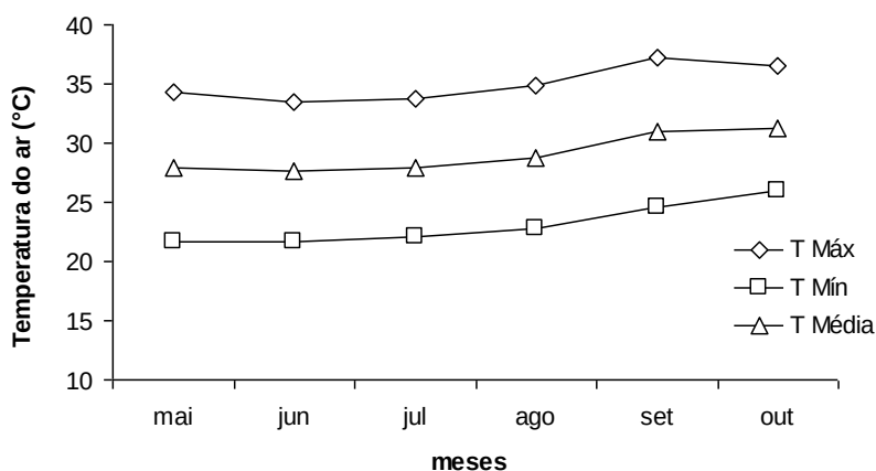
Figura 1. Variação mensal de temperatura máxima, média e mínima do ar no período experimental. Colatina-ES, 2009.
