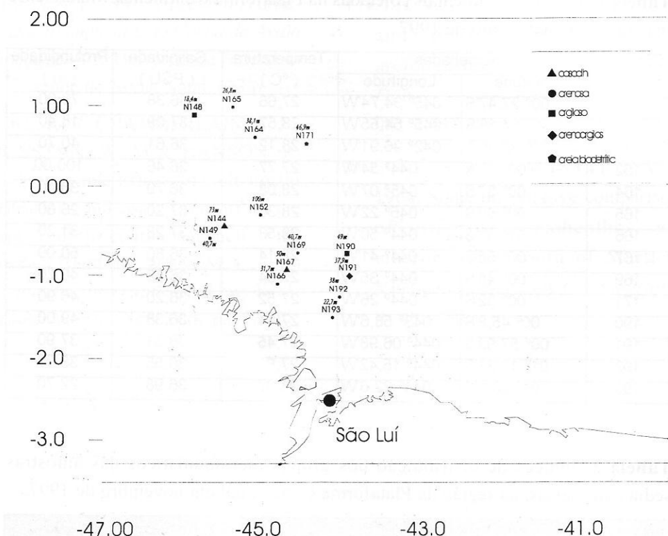
Figura 1. Tipos de fundo constatados em novembro de 1997, para as estações estudadas.
