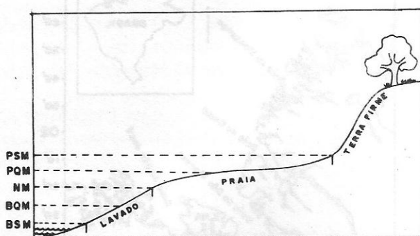
Figura 3 - Fisiografia de mesolitoral com lavado e praia na região do Golfo Maranhense. PSM - nível da preamar de sizígia; PQM - nível da preamar de quadratura; NM - nível médio da maré; BQM - nível da baixamar de quadratura; BSM - nível da baixamar de sizígia.
