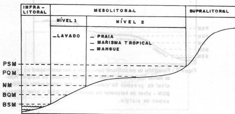
Figura 2 - Corte esquemático do mesolitoral mostrando a distribuição das unidades naturais nos níveis 1 e 2. PSM - nível da preamar de sizígia; PQM - nível da preamar de quadratura; NM - nível médio da maré; BQM - nível da baixamar de sizígia; BSM - nível da baixamar de sizígia.
