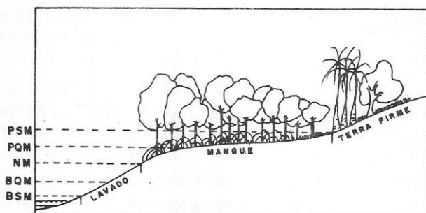
Figura 4 - Fisiografia de mesolitoral com lavado e mangue na região do Golfo Maranhense. PSM - nível da preamar de sizígia; PQM - nível da preamar de quadratura; NM - nível médio da maré; BQM - nível da baixamar de quadratura; BSM - nível da baixamar de sizígia.
