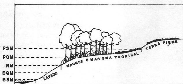
Figura 6 - Fisiografia de mesolitoral com lavado, mangue e marisma tropical na região do Golfo Maranhense. PSM - nível da preamar de sizígia; PQM - nível da preamar de quadratura; NM - nível médio da maré; BQM - nível da baixamar de quadratura; BSM - nível da baixamar de sizígia.
