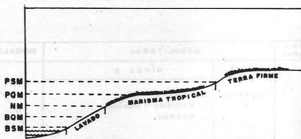
Figura 5 - Fisiografia de mesolitoral com lavado e marisma tropical na região do Golfo Maranhense. PSM - nível da preamar de sizígia; PQM - nível da preamar de quadratura; NM - nível médio da maré; BQM - nível da baixamar de quadratura; BSM - nível da baixamar de sizígia.
