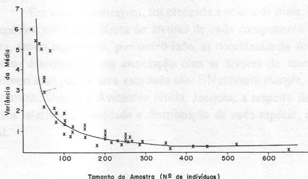
FIGURA Nº 1 - Variância da média em função do número de indivíduos mensalmente amostrados do camarão vermelho, Penaeus aztecus subtilis Pérez Farfante, 1967, capturados em Tutóia (Maranhão), durante os meses de julho de 1978 a setembro de 1979.
