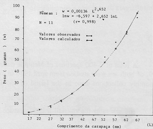
FIG. Nº 14 - Regressão do Peso total (g) sobre o comprimento da carapaça (mm) de Menippe nodifrons Stimpson, 1859, na Costa do Estado do Maranhão.
