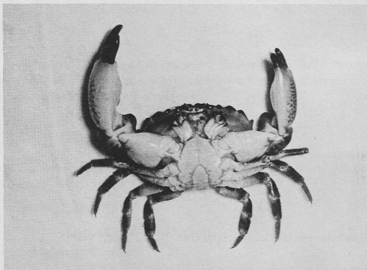
FIGURA N° 08 – Exemplar macho de siri-guajá Menippe nodifrons Stimpson, 1859.
