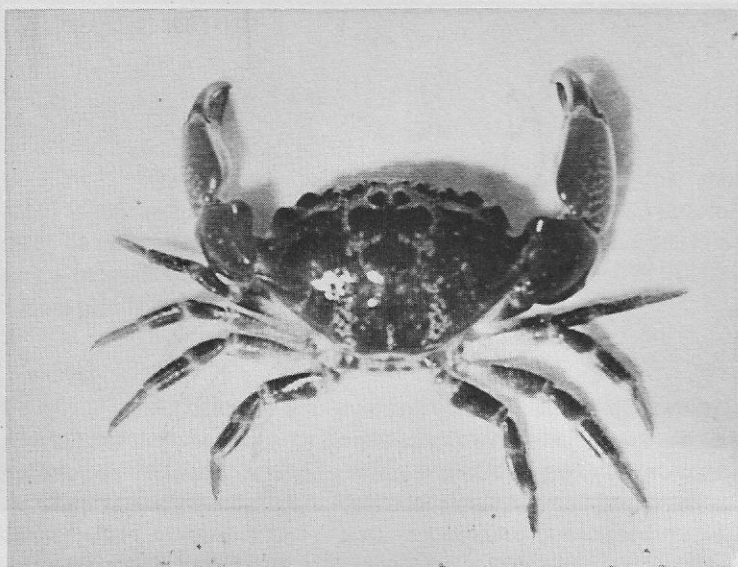
FIGURA N° 07 – Siri-guajá Menippe nodifrons Stimpson, 1859.
