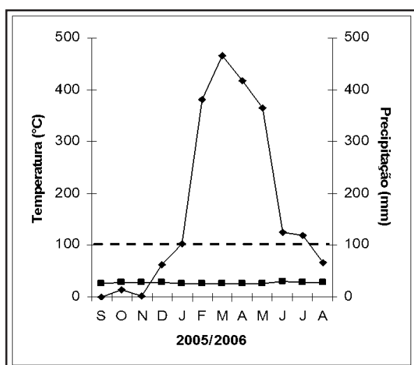
Figura 2. Diagrama climático baseado nos valores de temperatura (°C) e precipitação pluviométrica (mm) de setembro/2005 a agosto/2006. Dados provenientes da estação meteorológica de Tracuateua (INMET), Tracuateua – Pará.
