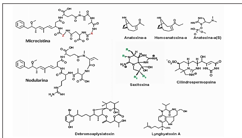
Figura 1. Estruturas químicas das principais cianotoxinas (desenhado com auxílio do software BKchem® 0.13.0). Fonte: Bortoli & Pinto (2015).
