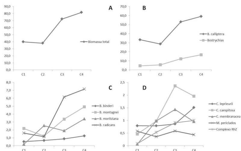
Figura 2. Variação da biomassa algácea (g.m -2 ) em valores totais das espécies de macroalgas ocorrentes em rizóforos de R. mangle L. na praia de Boa Viagem, São José de Ribamar, MA. A) biomassa total. B) B. calliptera x "Bostrychias". C) Espécies de Bostrychia. D) Demais espécies ocorrentes.
