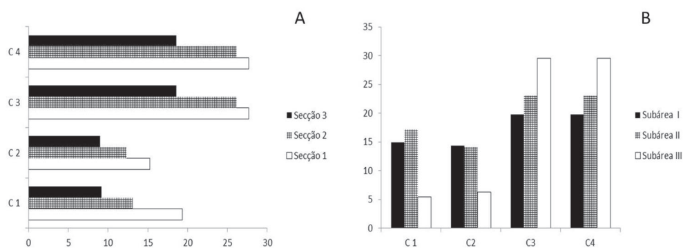
Figura 3. Variação da biomassa total (g.m -2 ) das macroalgas aderidas em rizóforos de R. mangle L. na praia de Boa Viagem, São José de Ribamar, MA. A) Biomassa por secção de rizóforo; B) Biomassa por subárea de transecto.
