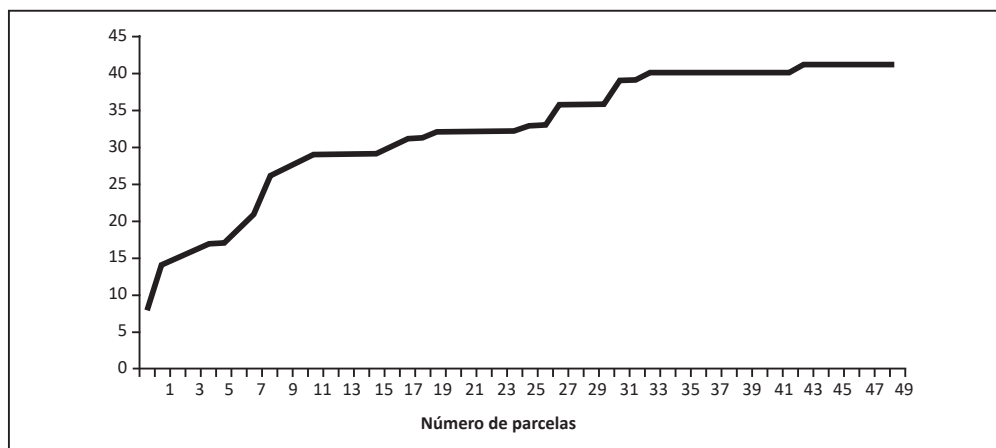
Figura 3. Curva de acumulação de espécies observadas em 50 parcelas (50 m²) amostradas na Praia de São Marcos, São Luís, Maranhão.
