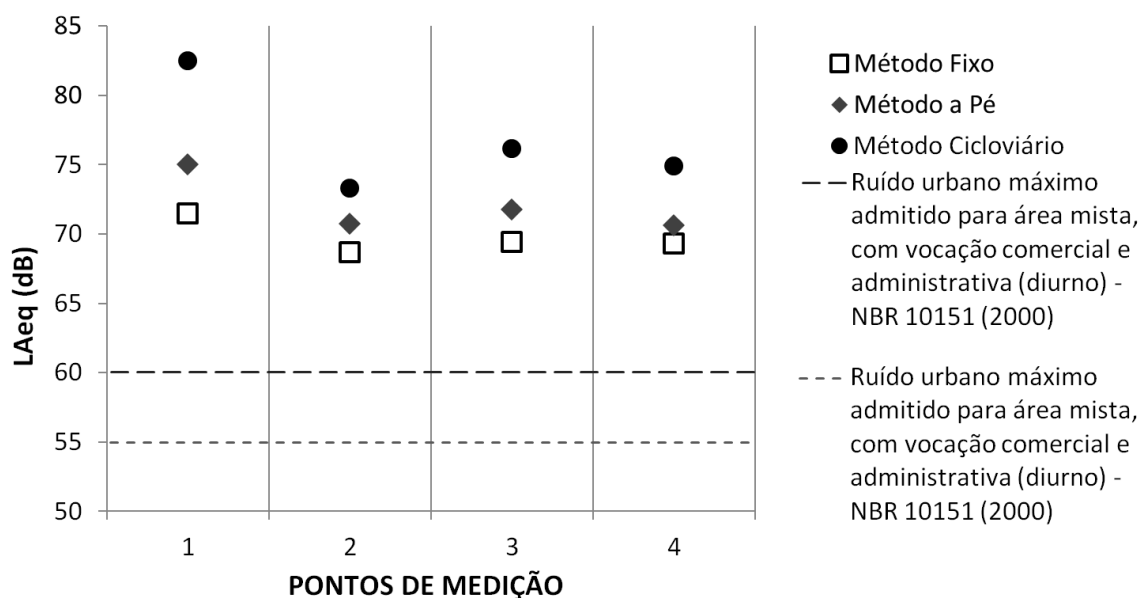
Fig. 5 - Comparação entre os dados medidos pelo Método Fixo, método do pedestre, método ciclístico, e determinações da NBR 10151.
