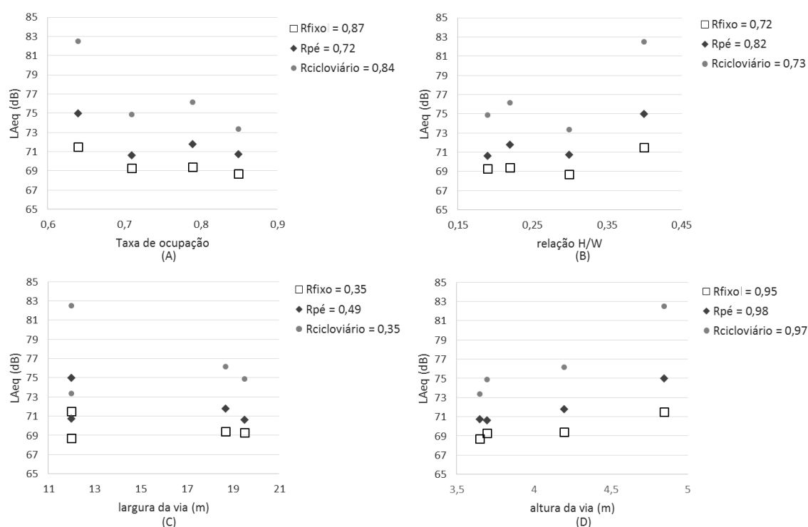
Fig. 6 – Relações entre parâmetros geométricos urbanos e os níveis de pressão sonora considerando: (A) Taxa de Ocupação; (B) Relação H/W; (C) Largura da via; (D) Altura da via
